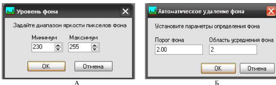
Рис. 3. Вид диалоговых окон «Уровень фона» (А) и «Автоматическое удаление фона» (Б)
