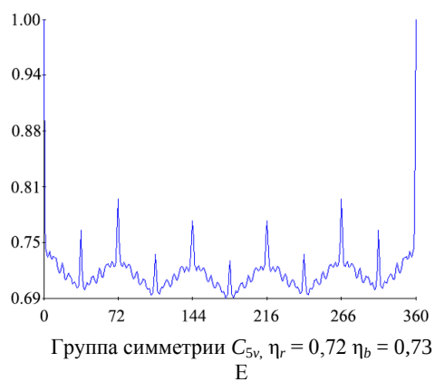
Рис. 3.19. Симметрологические характеристики диатомовых водорослей: А, В, Д – внешний вид; Б, Г, Е – симметрограммы. По оси ординат – степень инвариантности поворотной псевдосимметрии \eta_r (отн. ед.), по оси абсцисс – градусы поворота
