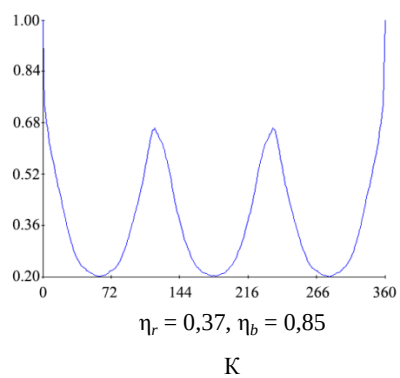
Рис. 3.23. Симметрологические характеристики скелета радиолярий отряда Radiiformata (Afanasieva et Amon, 2005). Изображения ставраконных радиолярий заимствованы из обсуждаемой работы Афанасьевой и Амон (2014). На графиках по оси ординат – степень инвариантности поворотной псевдосимметрии \eta_r (отн. ед.), по оси абсцисс – градусы поворота
