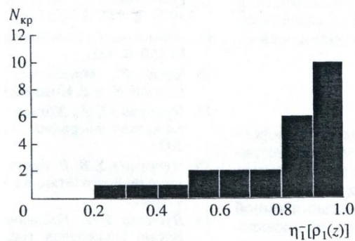
Рис. 4. Распределения числа кристаллов N_{кр} с известными значениями пироккоэффициентов по величине центросимметричности их функции \rho_1(z)
