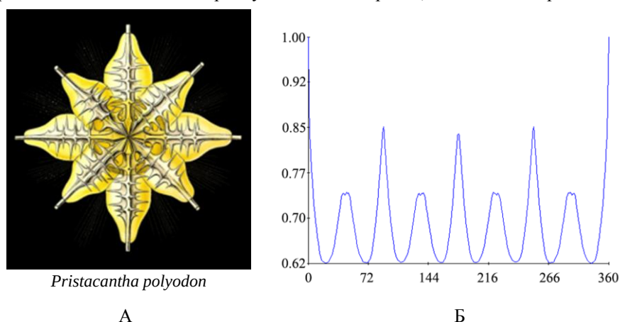
Рис. 3.22. Симметрологические характеристики радиолярии Pristacantha polyodon . А – внешний вид, Б – симметрограмма; группа симметрии C_{4v} , \eta_r = 0,68 , \eta_b = 0,85 . По оси ординат – степень инвариантности поворотной псевдосимметрии \eta_r (отн. ед.), по оси абсцисс – градусы поворота
