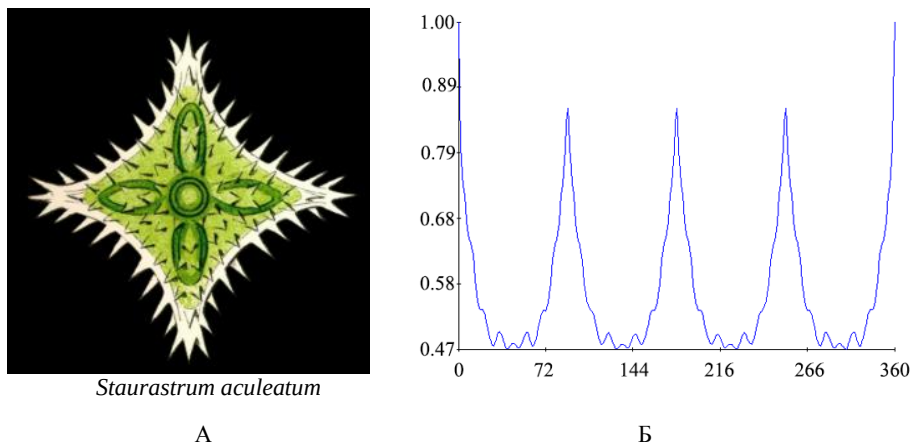
Рис. 3.17. Симметрологические характеристики водорослей Staurastrum aculeatum : А – внешний вид, Б – симметрограмма; группа симметрии C_{4v} ; \eta_r = 0,57 , \eta_b = 0,86 . По оси ординат – степень инвариантности поворотной псевдосимметрии \eta_r (отн. ед.), по оси абсцисс – градусы поворота
