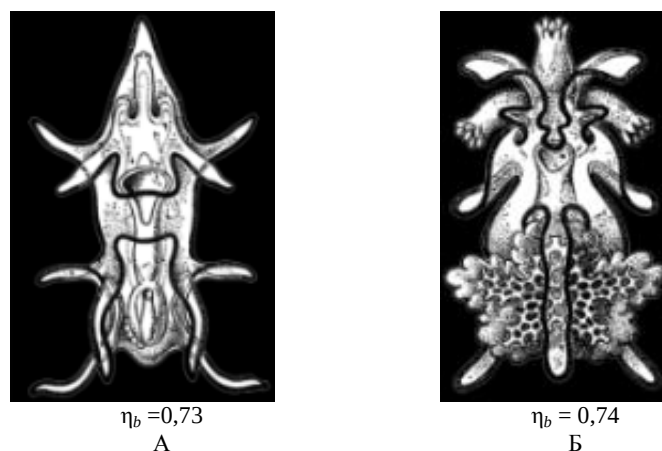
Рис. 3.32. Брахиоларии на разных стадиях развития и их симметрологические показатели. Группа симметрии C_s
