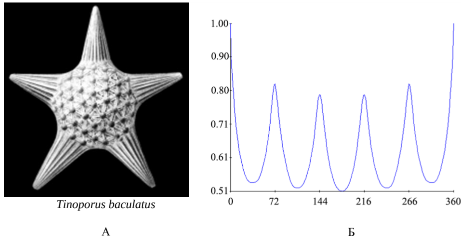
Рис. 3.20. Симметрологические характеристики фораминиферы Tinoporos baculatus : А – внешний вид, Б – симметрограмма; группа симметрии C_{5v} , \eta_r = 0,62 , \eta_b = 0,82 . По оси ординат – степень инвариантности поворотной псевдосимметрии \eta_r (отн. ед.), по оси абсцисс – градусы поворота
