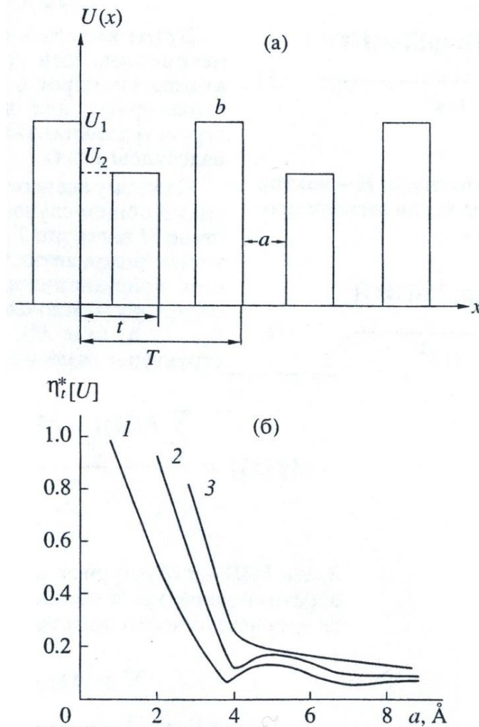
Рис. 3. Одномерный потенциал с трансляционной псевдосимметрией (а) и графики зависимости \eta_t^*[U] от расстояния a между барьерами для различных значений ширины потенциальных барьеров b в одномерной модели Кронига–Пенни (б): 1 – b = 1 \text{ \AA} , 2 – b = 2 \text{ \AA} , 3 – b = 3 \text{ \AA}
