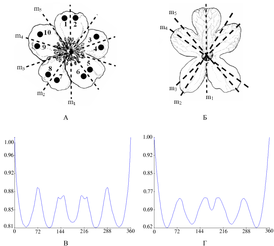
Рис. 3.3. Анализ поворотной псевдосимметрии. А, Б – схемы венчика актиноморфного и зигоморфного цветков; В, Г – соответствующие симметрограммы. По оси ординат – степень инвариантности поворотной псевдосимметрии \eta_r (отн. ед.), по оси абсцисс – градусы поворота
