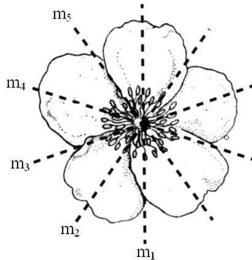
Рис. 2.7. Схема актиноморфного цветка из работы Donoghue et al. (1998), m_1...m_5 – плоскости симметрии
