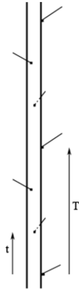
Рис. 2.3. Пример спирального листорасположения, описываемого винтовым поворотом третьего порядка
