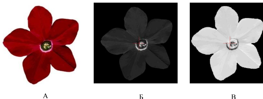
Рис. 9. Внешний вид цветка душистого табака: А – без изменений; Б – при загрузке изображения в программу и его автоматическом переводе из цветного изображения в изображение с 256 градациями серого; В – вид цветка при применении операции инверсии цвета и повторной обработки фона
