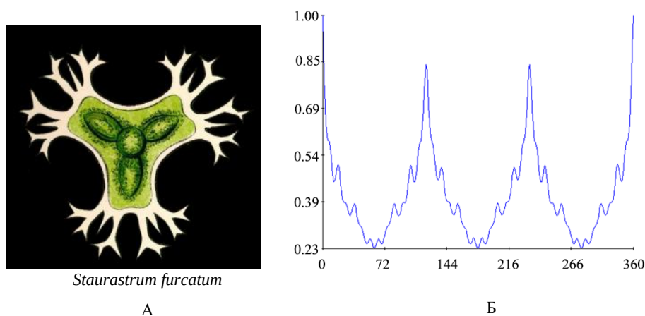
Рис. 3.16. Симметрологические характеристики водорослей Staurostrum furcatum :
