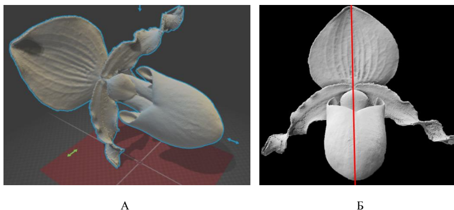
Рис. 4.19. Орхидея башмачок ( Cypripedium ): А – изображение 3D-модели цветка, формируемое при сканировании; Б – фронтальное изображение 3D-модели цветка, красная линия – плоскость зеркальной симметрии, перпендикулярна плоскости изображения
