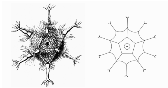
Рис. 2. Скелеты Circogonia icosahedra (слева, по Э. Геккелю) и C. dodecahedra (справа, по Д.Д. Мордухай-Болтовскому), геометрически дуальные простейшему фуллерену – додекаэдру
