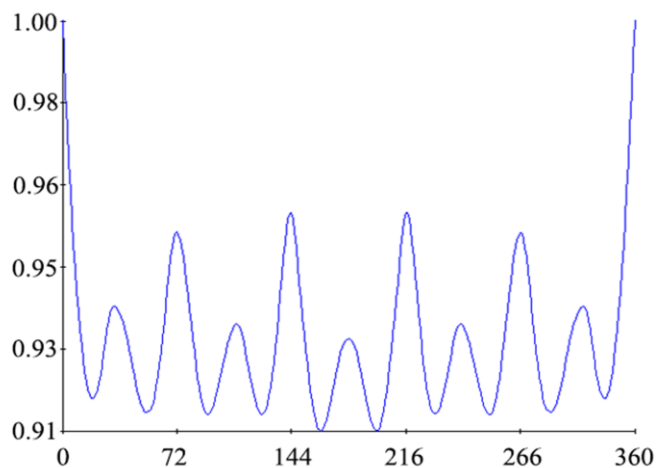
Рис. 3.35. Симметрограмма венчика цветка примулы P. x polyantha культурной формы Lutea . По оси ординат – степень инвариантности поворотной псевдосимметрии \eta_r (отн. ед.), по оси абсцисс – градусы поворота
