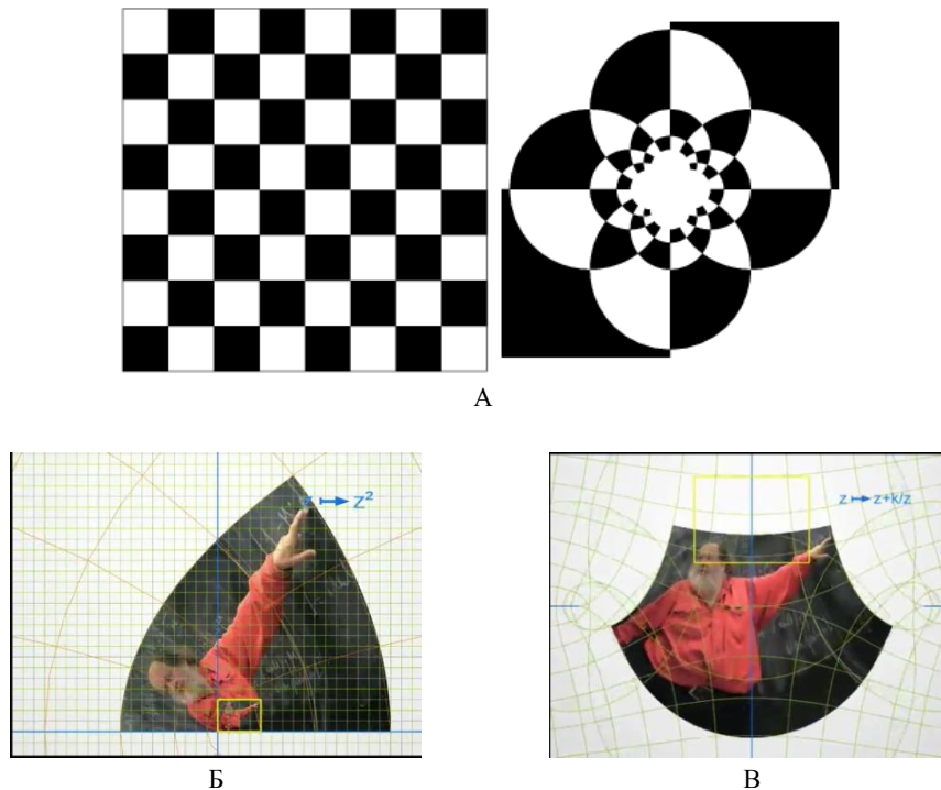
Рис. 1.6. Примеры конформных отображений:
