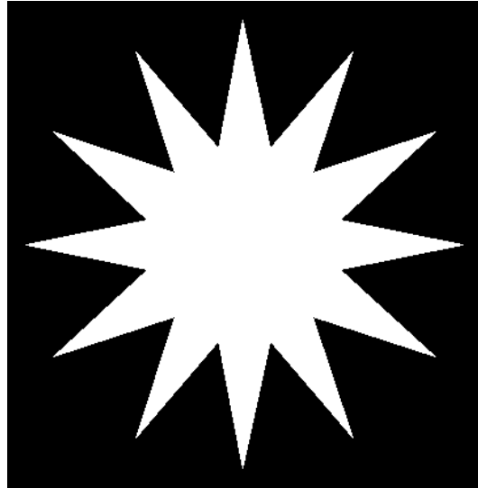
Рис. 3.1. Пример изображения объекта (12-лучевой звезды) с осью поворотной симметрии 12-го порядка
