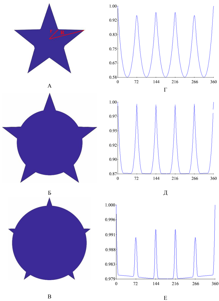
Рис. 3.11. Форма модельных звезд и соответствующие симметрограммы при разных соотношениях перррадиуса и интеррадиуса ( R/r ). На Г, Д, Е по оси ординат – степень инвариантности поворотной псевдосимметрии \eta_r (отн. ед.), по оси абсцисс – градусы поворота
