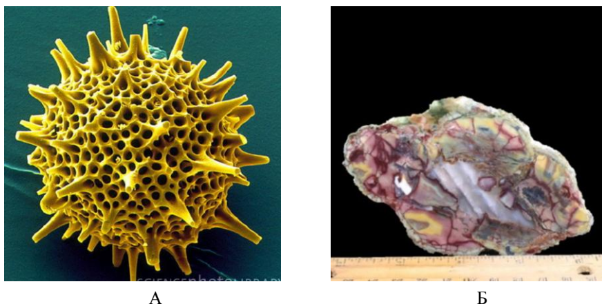
Рис. 3.21. А – скелет радиолярии, Б – яшма
