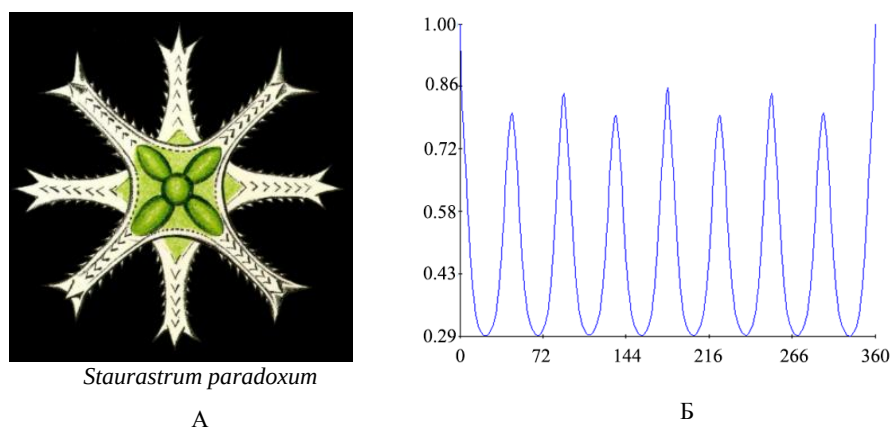
Рис. 3.18. Симметрологические характеристики водорослей Staurastrum paradoxum : А – внешний вид, Б – симметрограмма; группа симметрии C_{4v} ; \eta_r = 0,48 , \eta_b = 0,83 . По оси ординат – степень инвариантности поворотной псевдосимметрии \eta_r (отн. ед.), по оси абсцисс – градусы поворота
