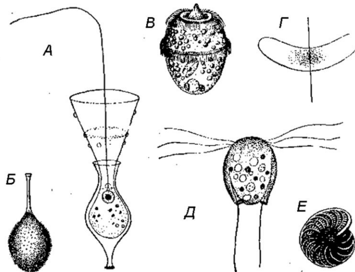
Рис. 4. Монаксонно-гетерополярные и двусторонне-симметричные простейшие:
