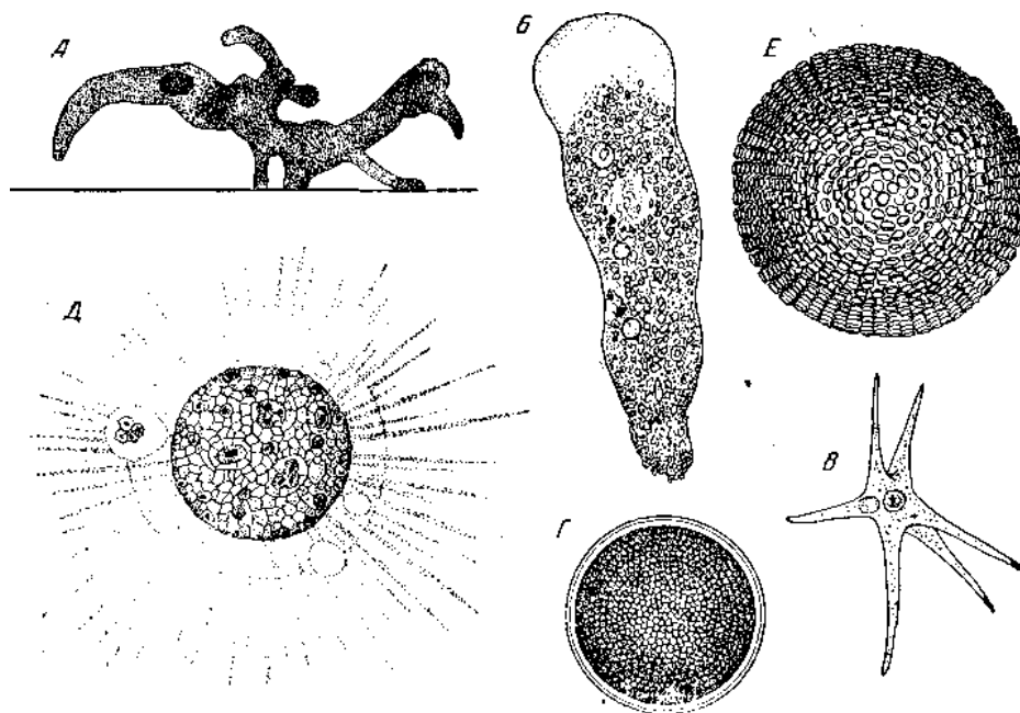
Рис. 2. Анаксонные и неопределенно полиаксонные простейшие:
