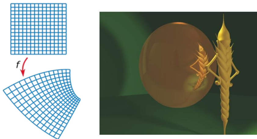
Рис. 1.3. Примеры конформного отображения
