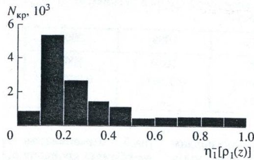
Рис. 5. Распределение кристаллов с группами симметрии из классов C_n и C_{nv} по величине \eta_1[\rho_1(z)] (по данным Кембриджского банка данных кристаллических структур 2004 г.)
