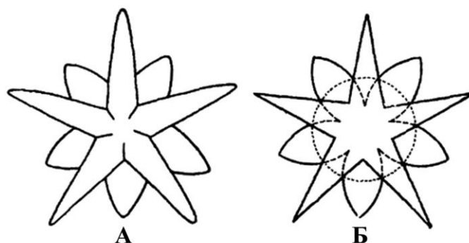
Рис. 3.7. Примеры конформной симметрии (Петухов, 1981). А, Б — цветок и схема, поясняющая конформное отображение цветка
